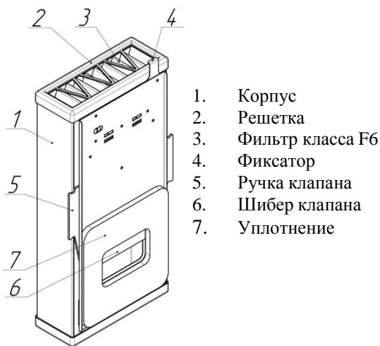
Рис. 3 Устройство шумоглушителя
